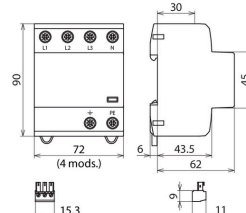
Beépítési méretek DSH TNS 255 FM
