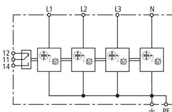
Kapcsolási rajz DSH TNS 255 FM
